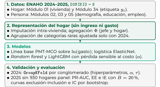
Figura 1: Flujo metodológico. y_i : pobreza oficial del hogar; \Phi : agregación de personas a hogar; \alpha : peso de la clase pobre en la pérdida; \tau : umbral de decisión; B : proporción de hogares seleccionados; EE e IE: errores de exclusión e inclusión.
